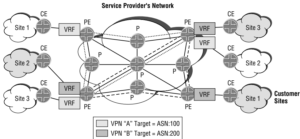
FIGURE 7.2 2547 bis terminology
